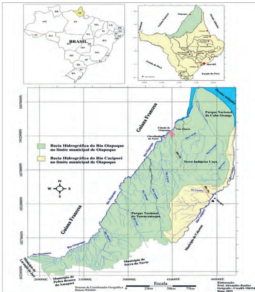
Figura 1: Localização da Bacia do Rio Oiapoque e seus afluentes da margem direita
