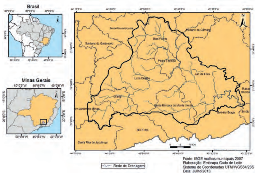
Figura 01: Bacia Hidrográfica do Rio do Peixe/MG, Sudeste do Brasil
