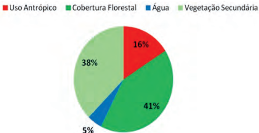
Gráfico 1: Classes na Bacia Hidrográfica do Rio Mojuí-PA
